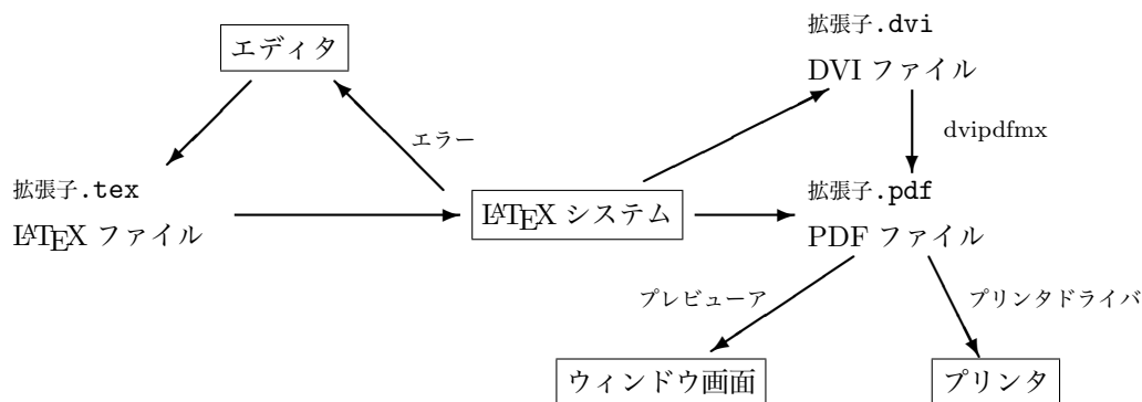
図 4.1 L A T E X システムにおける処理の流れ
