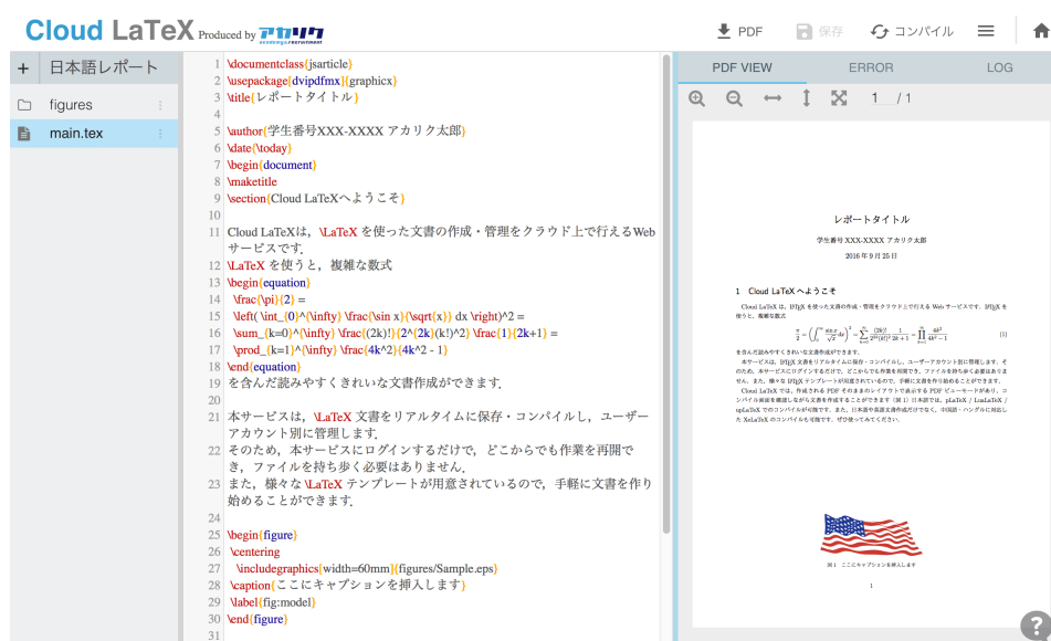
図 A.4 CloudLaTeX の日本語レポートの作成の様子。[テンプレートから作成] の日本語レポートは図の貼り込みをする例だ。
